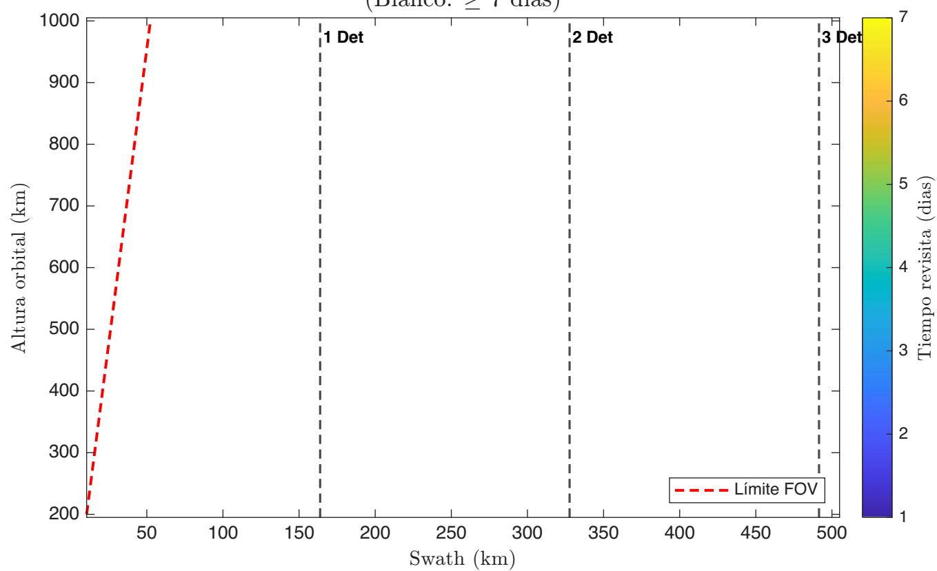
Tiempo Revisita - 2 Satellite(s); 1 Telescopio(s): Cassegrain; Detector 2 (Blanco: \geq 7 dias)
